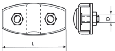
Galv. "DUPLEX SPECIAL" Pladewirelås
