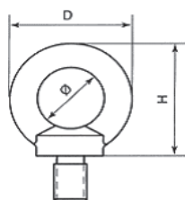
Syrefast, AISI 316 Øjebolt og Øjemøtrik DIN 580 & 582
