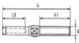
Syrefast, AISI 316 Gevindterminal S.S., AISI 316 Swage Stud
