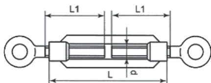
Syrefast, AISI 316 Bardunstrammer, Øje/Øje, DIN 1480
