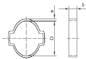
Rustfri, AISI 304 Øreklemme m/2 ører & 1 øre
